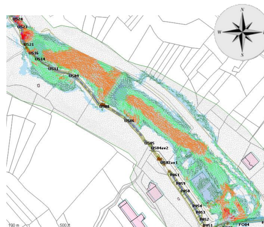
Figure 1 : Comparatif zone inondable Q100 amont pour l'état initial et l'état S6
