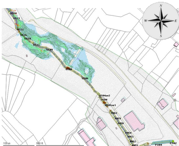
Figure 1 : Comparatif zone inondable Q10 pour l'état initial et l'état S6
